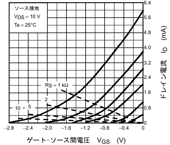
ID - VGS
